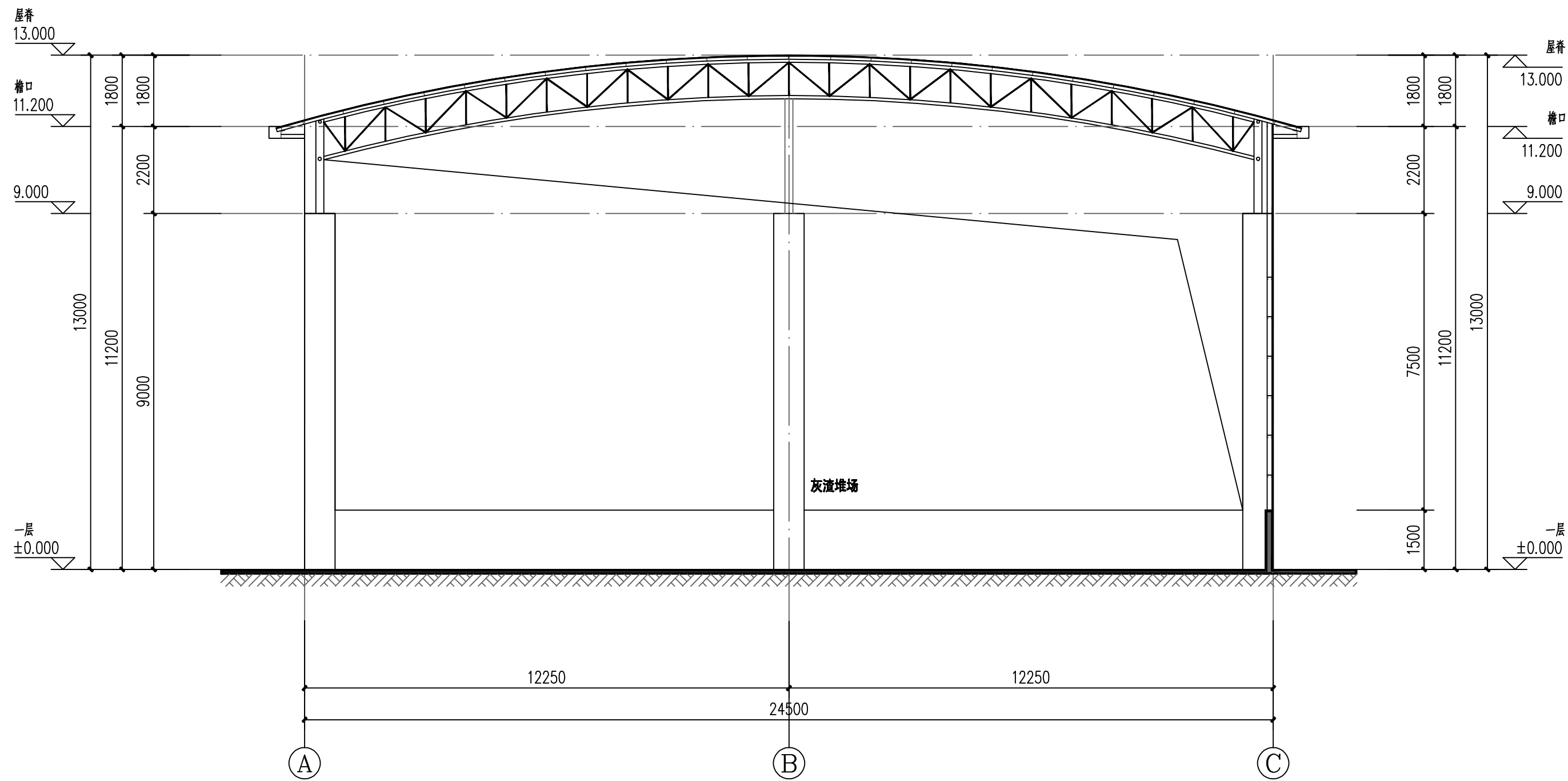
1-1剖面图 1:100
