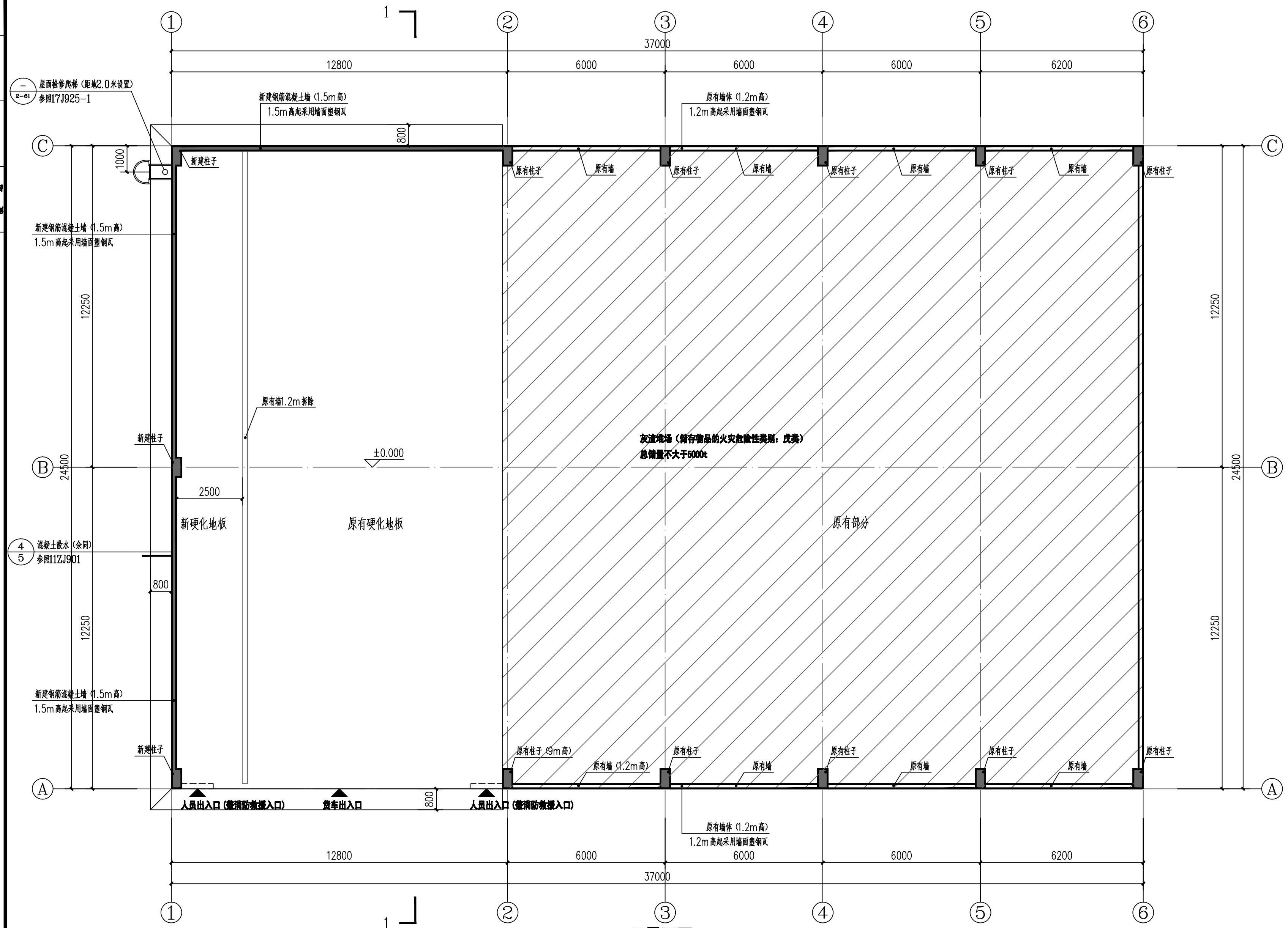
一层平面图 1:100
