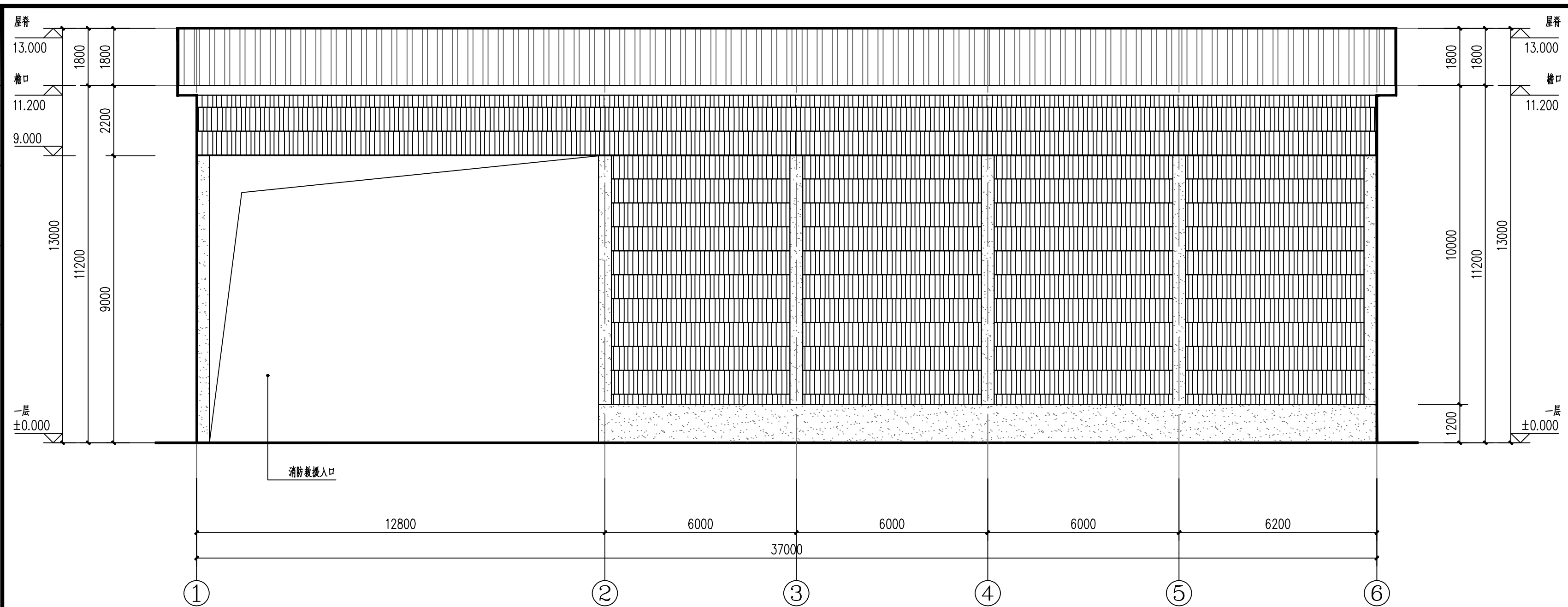
①轴~⑥轴立面图 1:100
