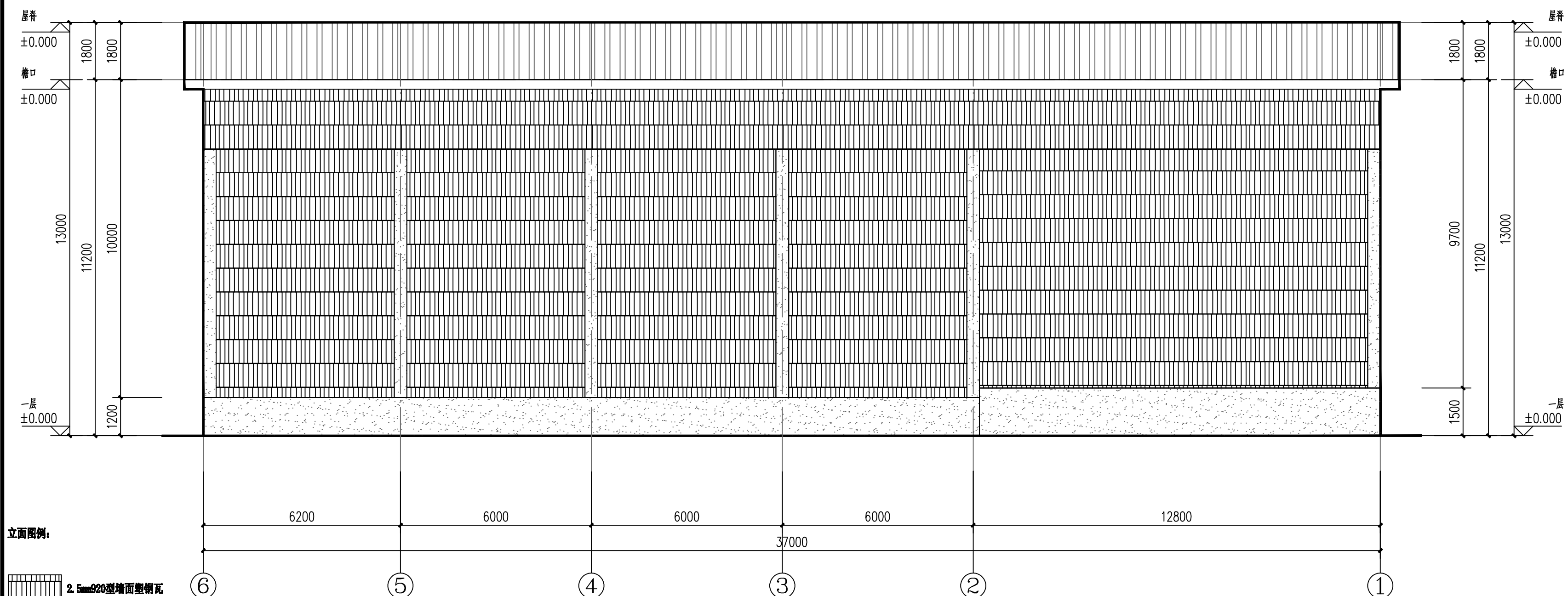
⑥轴~①轴立面图 1:100
