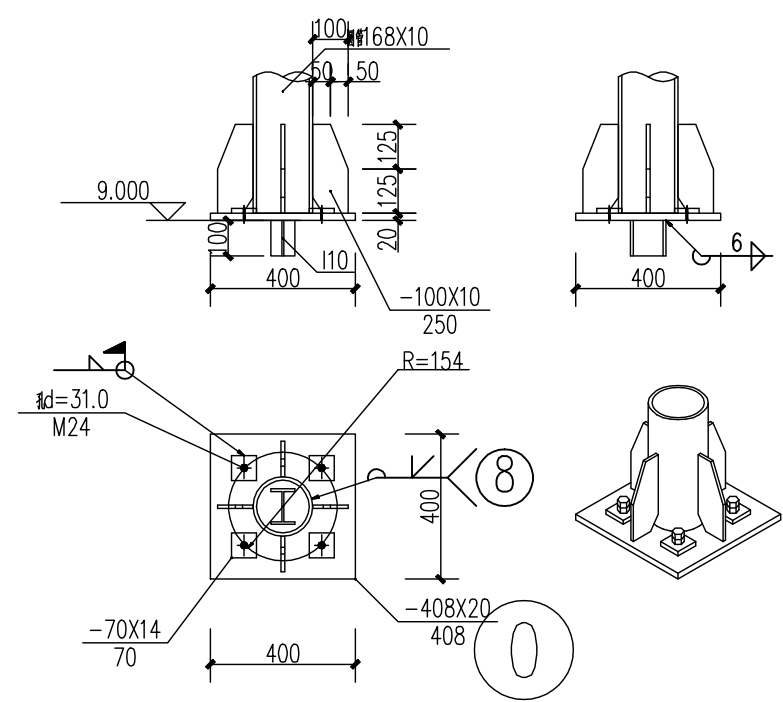
柱脚大样图
