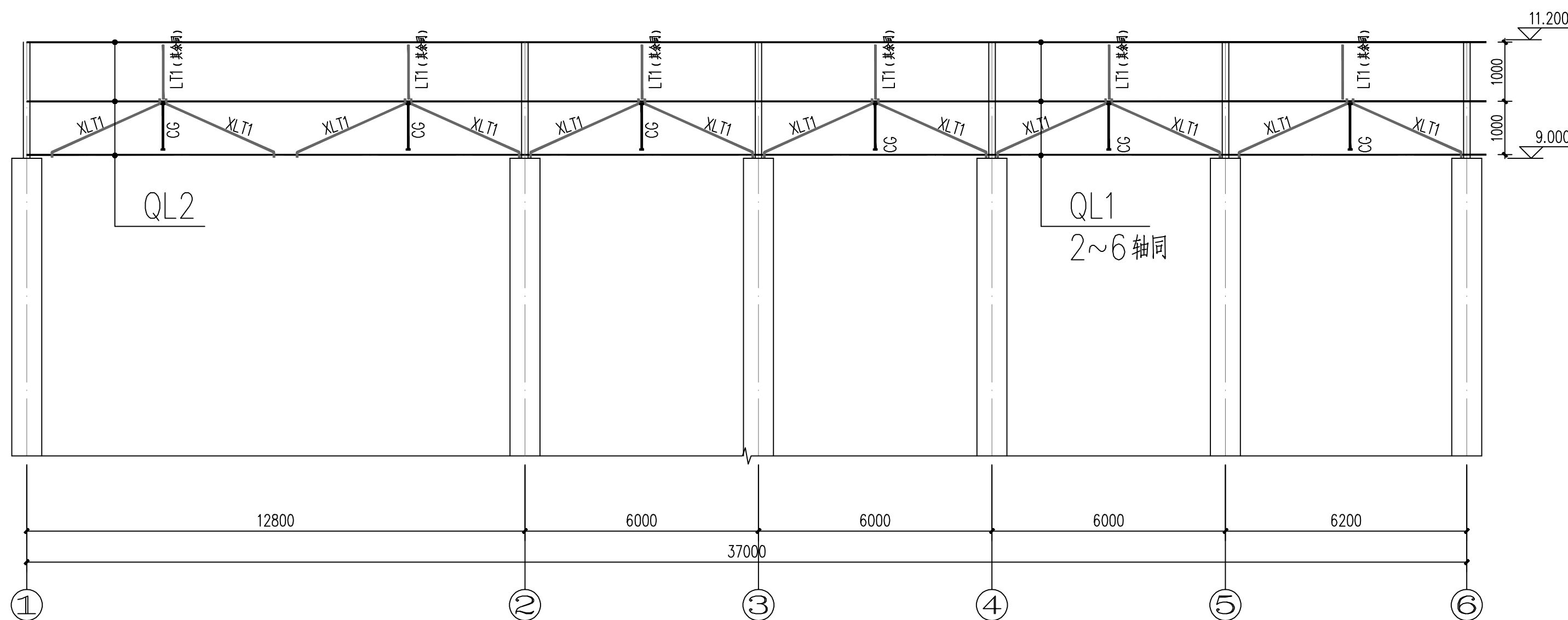
A、D轴墙面檩条
