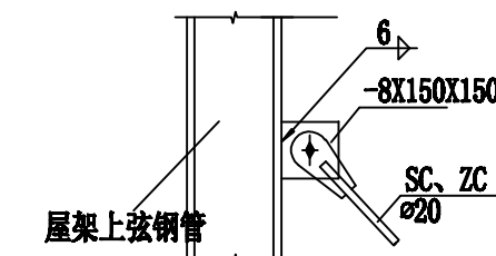
SC、ZC连接节点大样图
