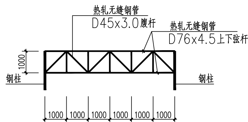
纵向支撑大样
