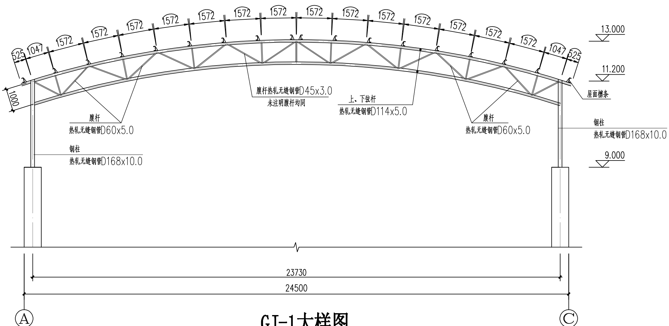
GJ-1大样图
