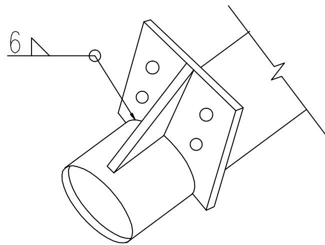
檯托大样图
