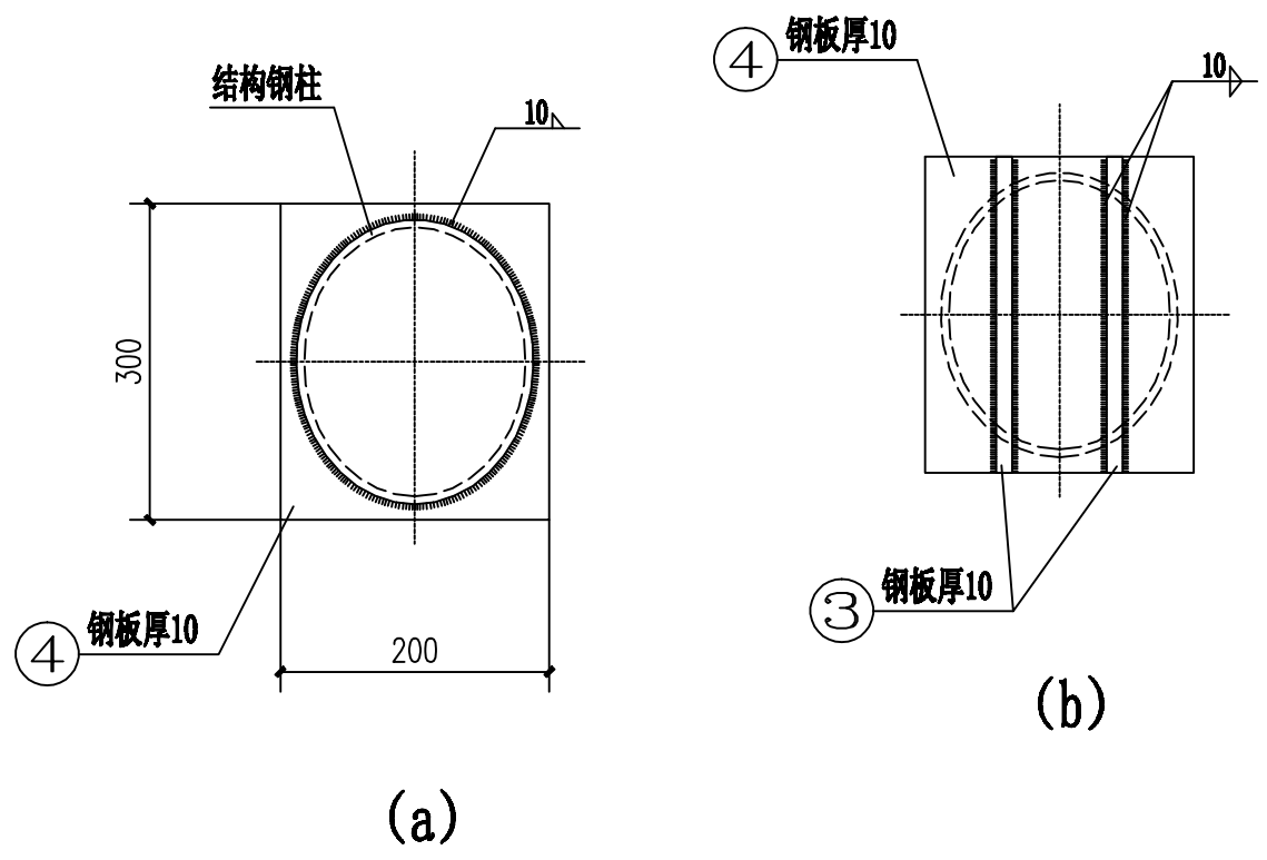
柱顶连接节点详图1
