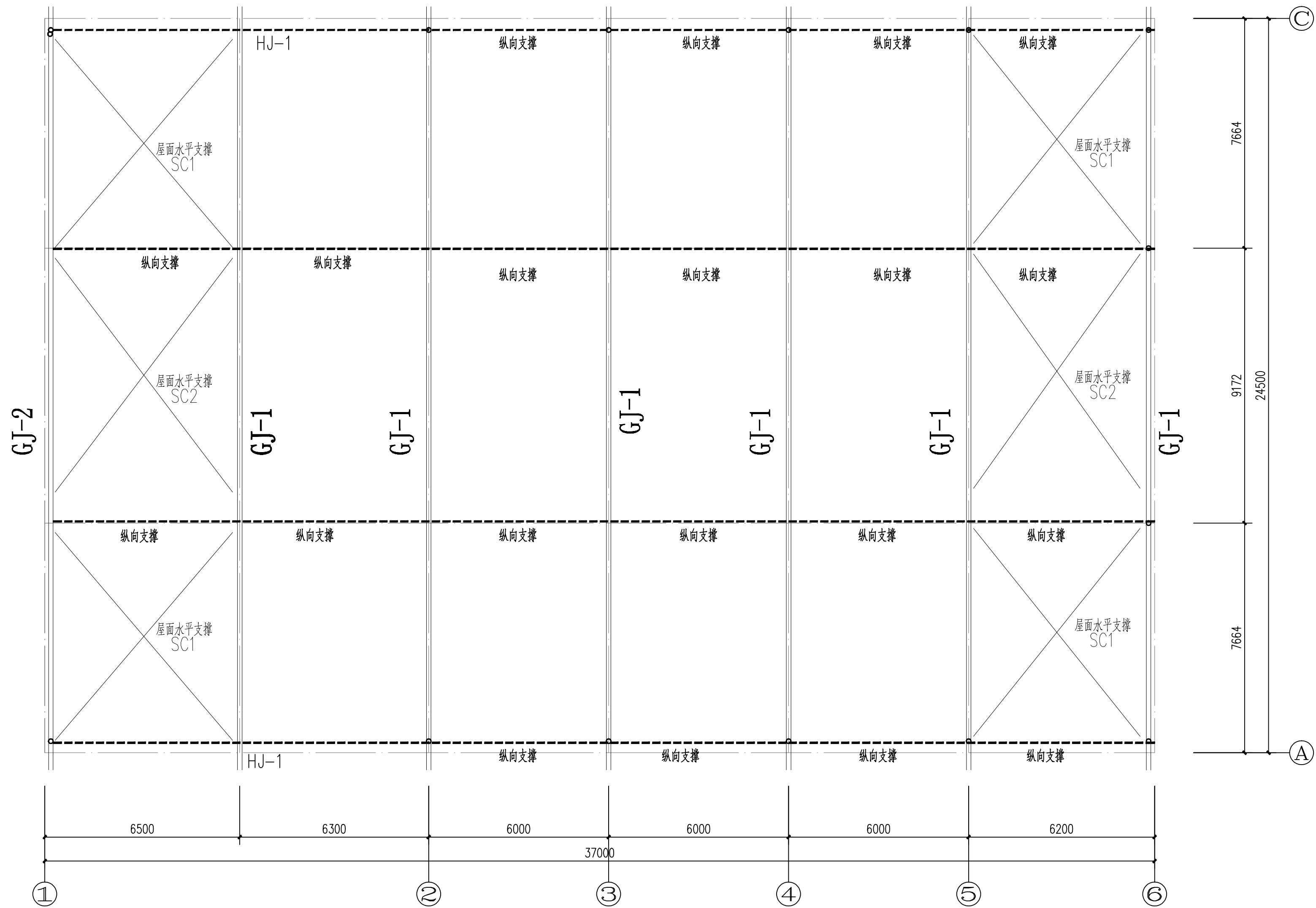
钢屋架及支撑布置图
