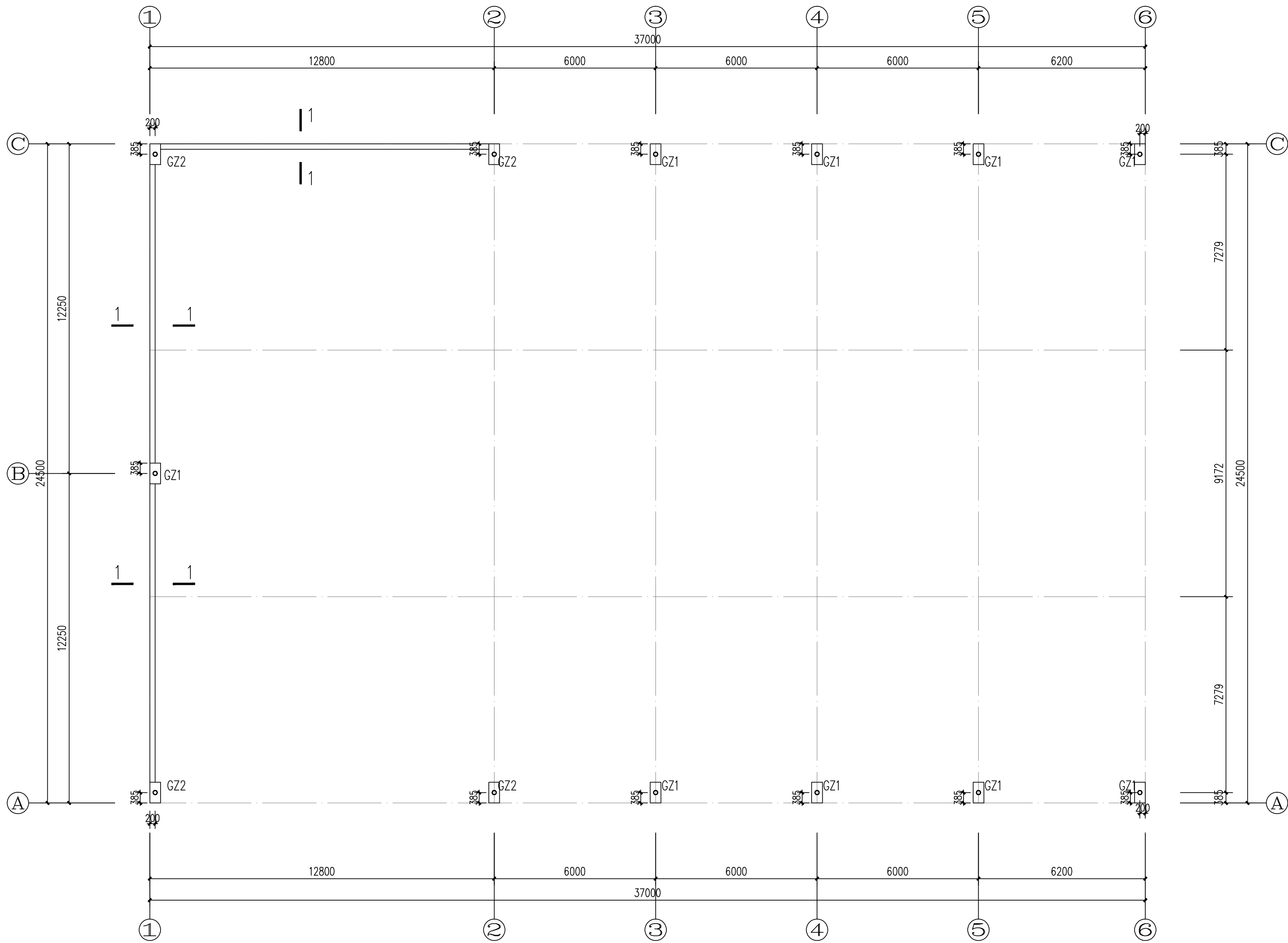
钢柱平面布置图
