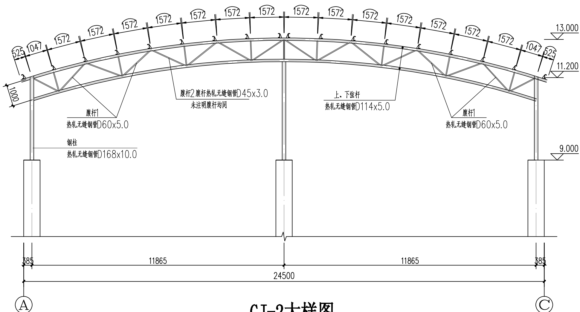
GJ-2大样图
