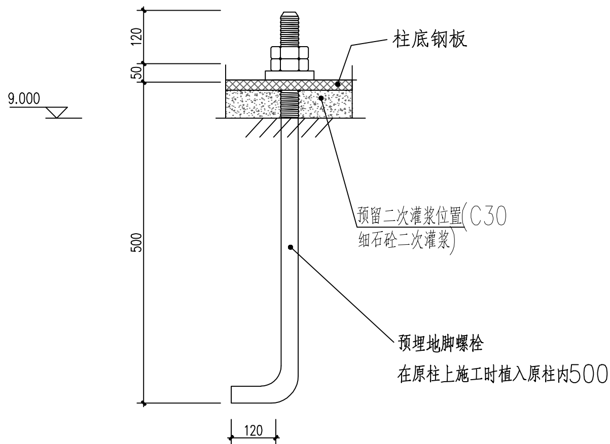
M24柱脚锚栓详图
