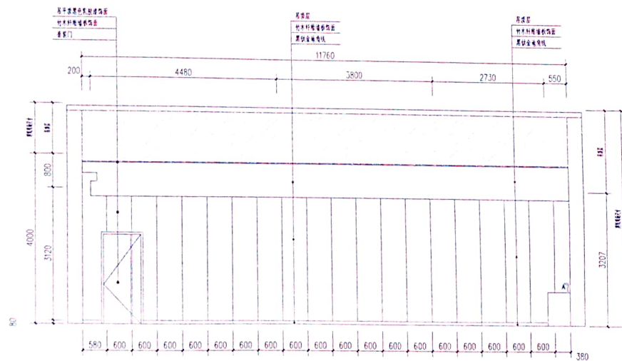
就餐区B立面 1:100
