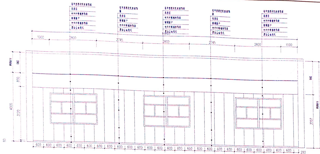
就餐区A立面 1:100
