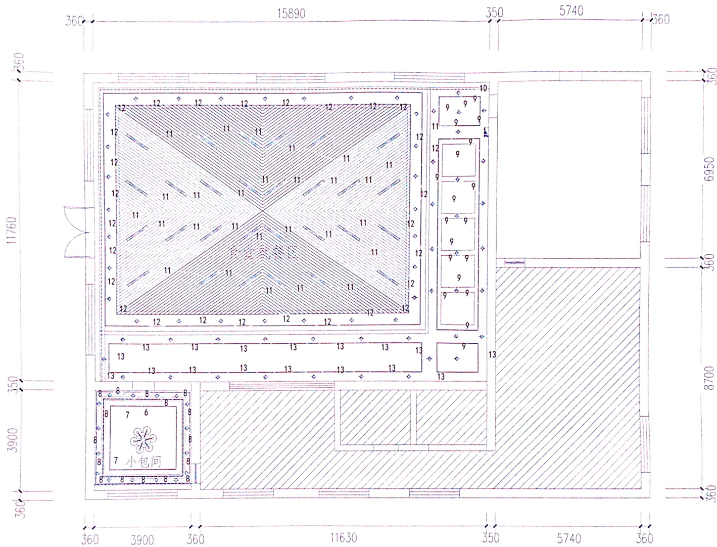
灯具布置图 1:100
