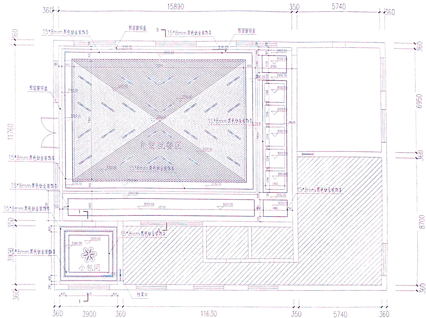
顶面吊顶图 1:100
