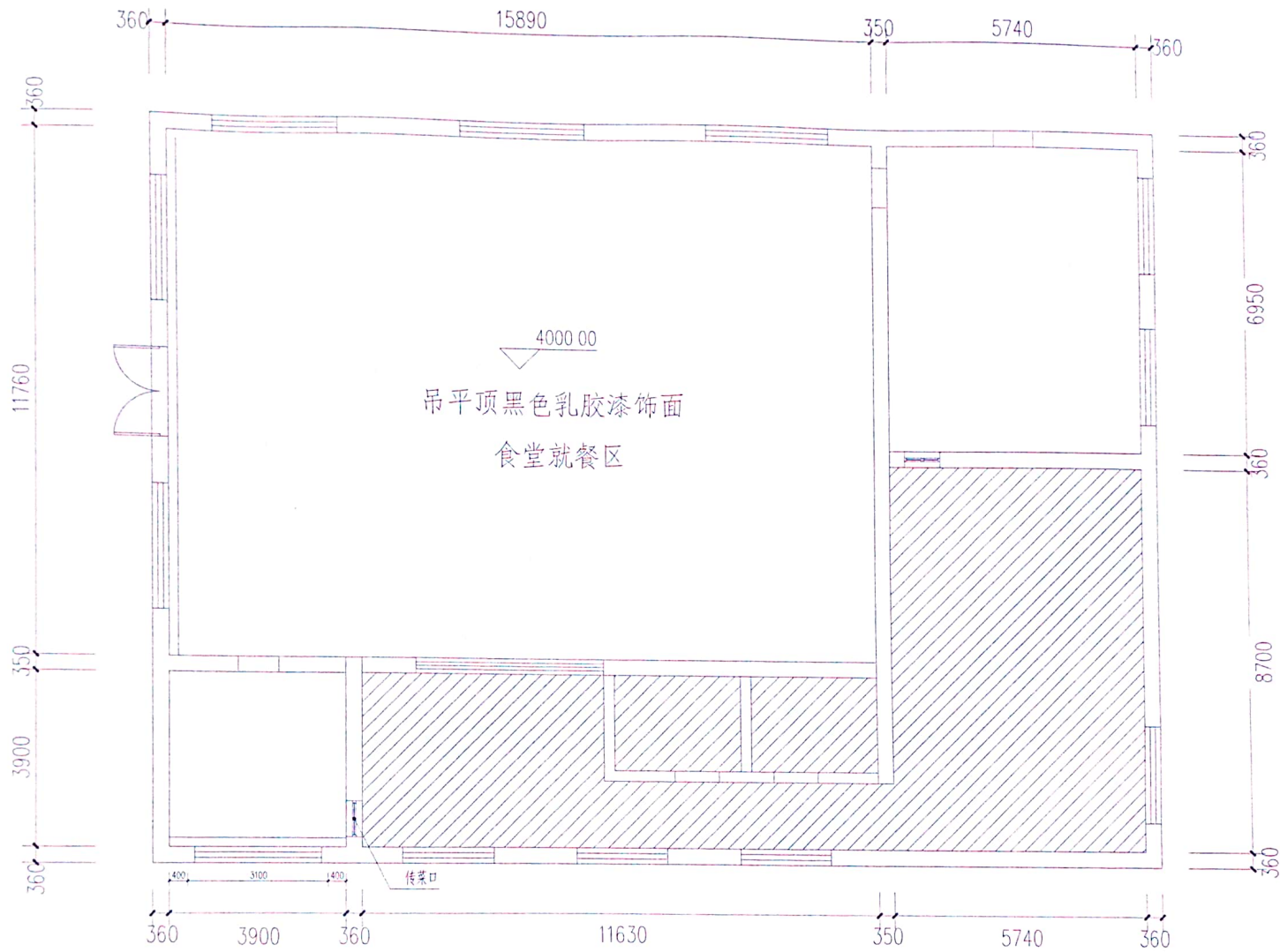
就餐区夹层吊顶图 1:100
