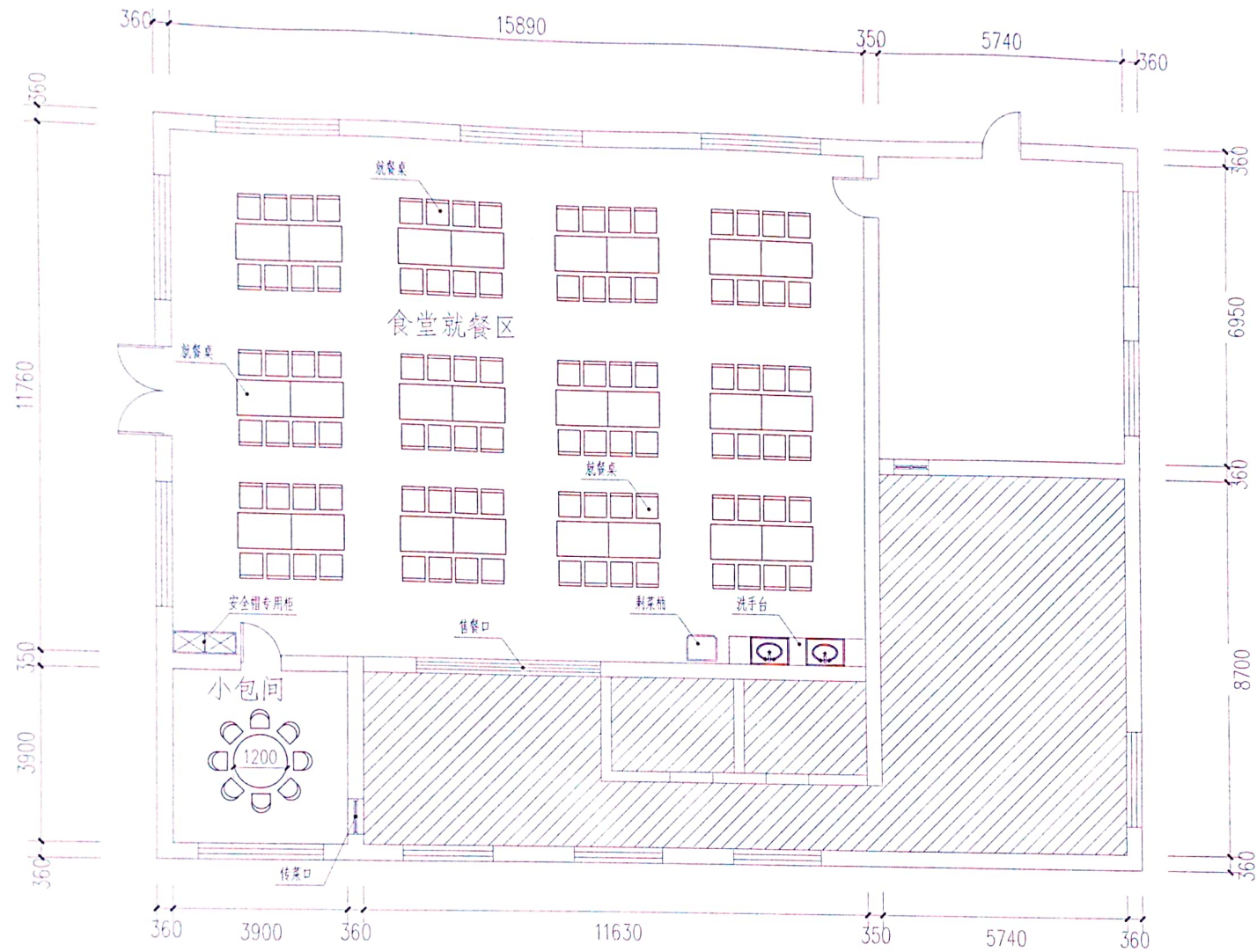
平面布置图 1:100
