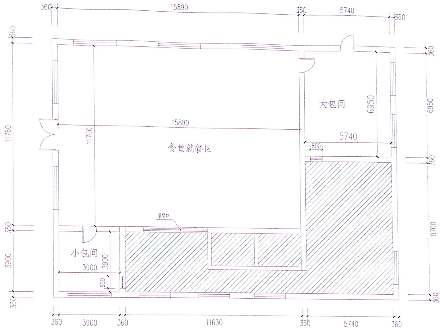
墙体改造图 1:100
