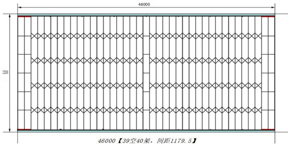
雨棚顶视图
