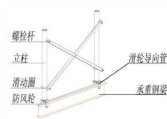
立柱伸缩架详图
