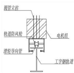
轨道结构详图
