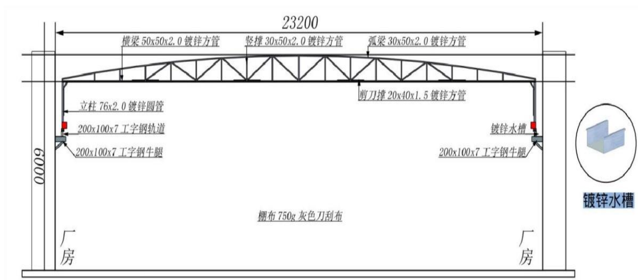
雨棚主梁框架示意图 宽度23.2米内高度6米
