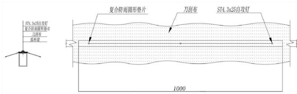
膜材安装方式详图
