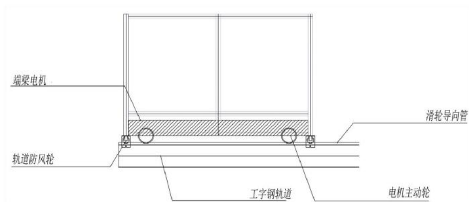
电机组装详图
